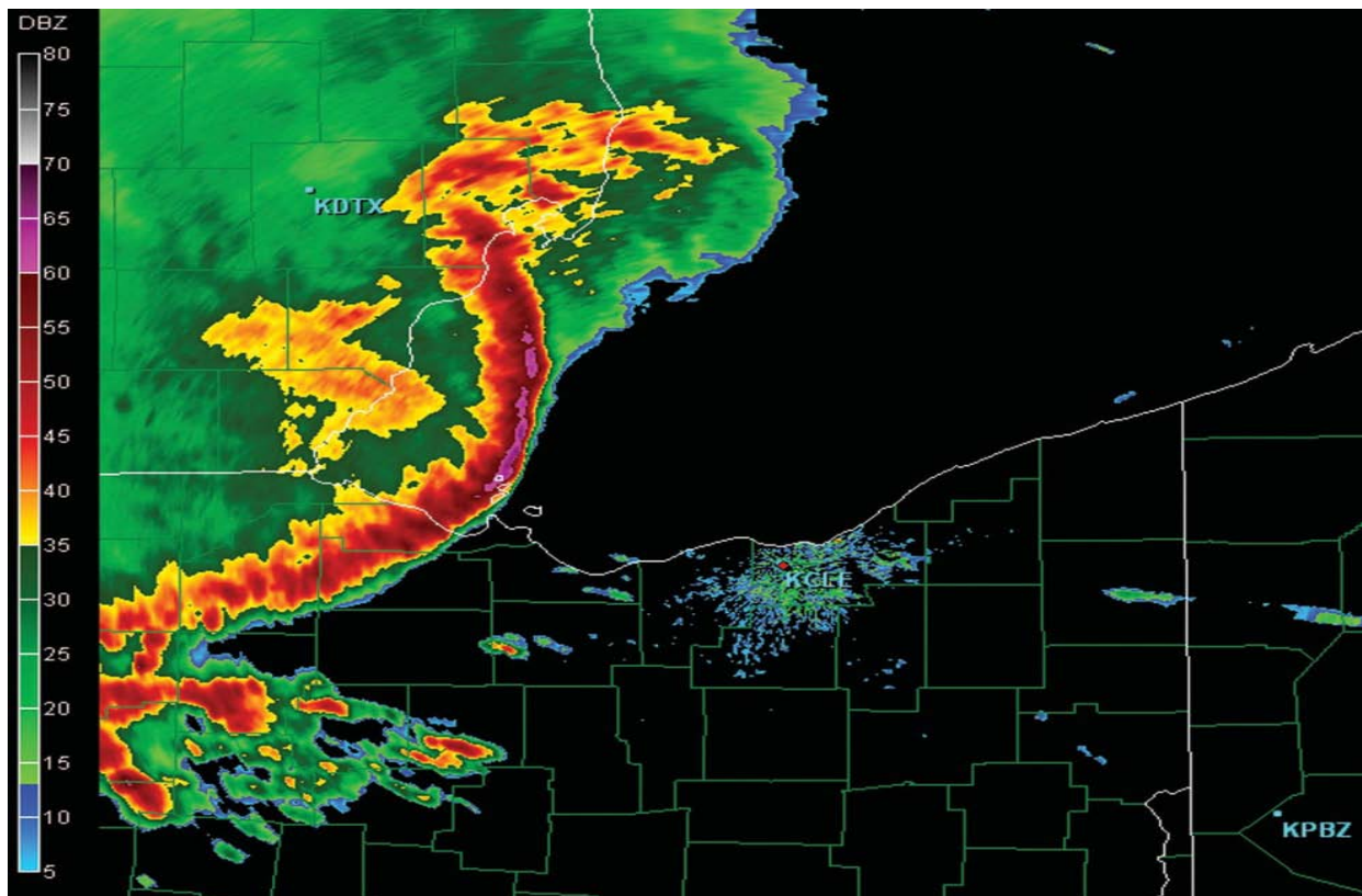
Una línea de turbonada severa, conocida como un derecho, en el noroeste de Ohio, el 21 de mayo de 2004.
