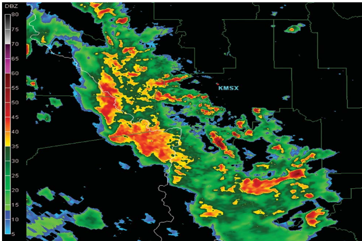
Este agrupamiento multicelular de tormentas produjo ráfagas de 60mph/97km/h en varias tormentas, resultando en ramas grandes quebradas en la parte oeste de Montana cerca de Missoula, Montana. La imagen viene del Radar Doppler del NWS/Missoula el 4 de junio de 2007.
