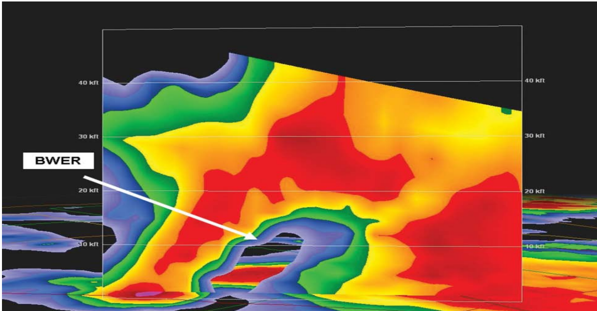
La Región de Eco Débil Acotada (REDA) indicada en una sección transversal del tornado en la Ciudad de Oklahoma el 3 de mayo de 1999.
