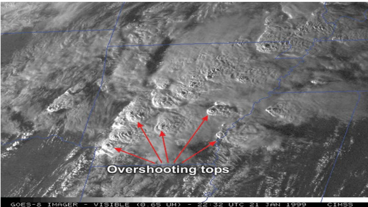
Una imagen de satélite visible indicando las cimas penetrantes sobre Arkansas el 21 de enero de 1999.
