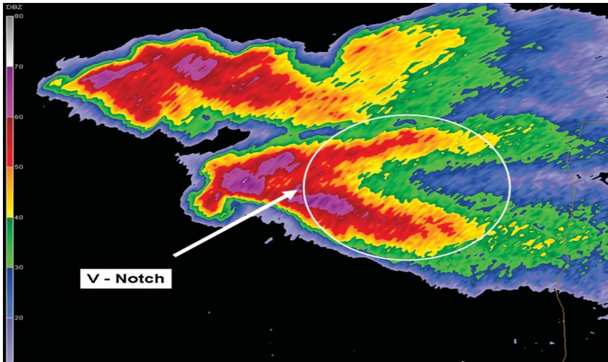
El Patrón en V en una tormenta supercelular el 24 de junio de 2008, del radar KLNK.
