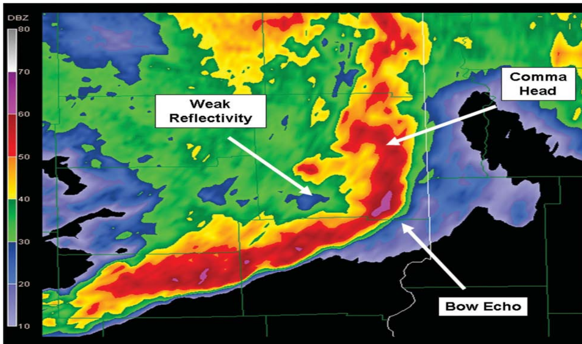
Los rasgos de radar de un eco en arco en el sudeste de Illinois el 3 de junio de 2008.
