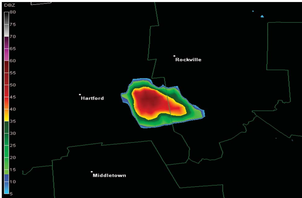
Una tronada de célula individual observada por el radar de Boston el 9 de junio de 2008.
