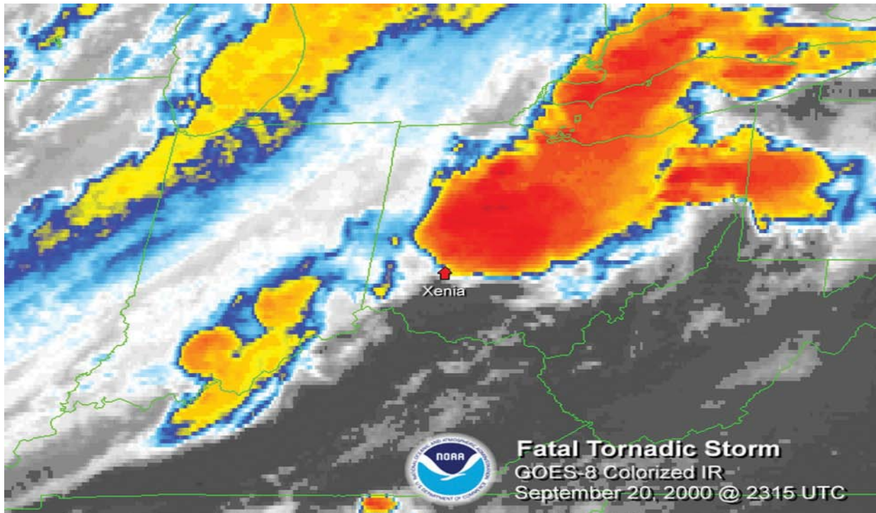
Una imagen infrarroja (IR) de una tronada que produjo un tornado cerca de Xenia, Ohio, el 20 de septiembre de 2000.
