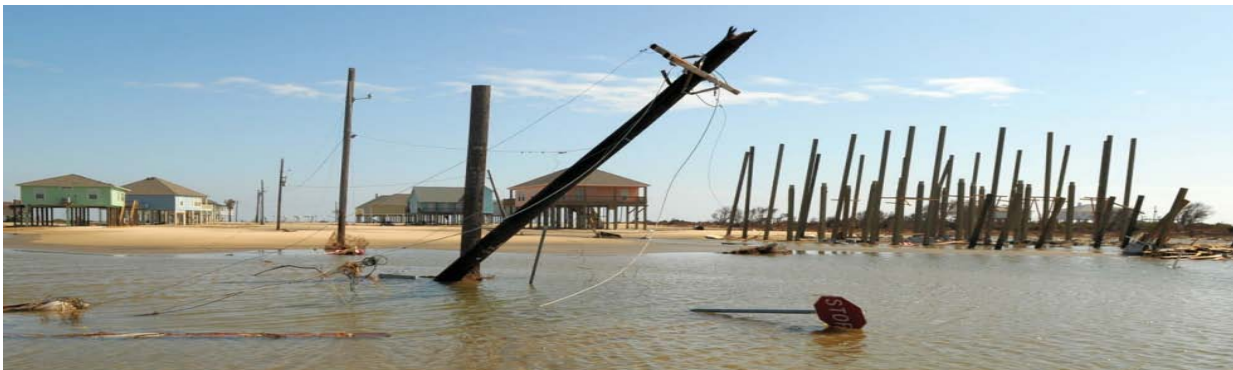
La Península Bolívar, Texas, el 20 de septiembre de 2008: Casas destruidas, escombros y líneas eléctricas caídas como resultado del huracán Ike. Fotografía por cortesía de Jocelyn Agostino, FEMA.
