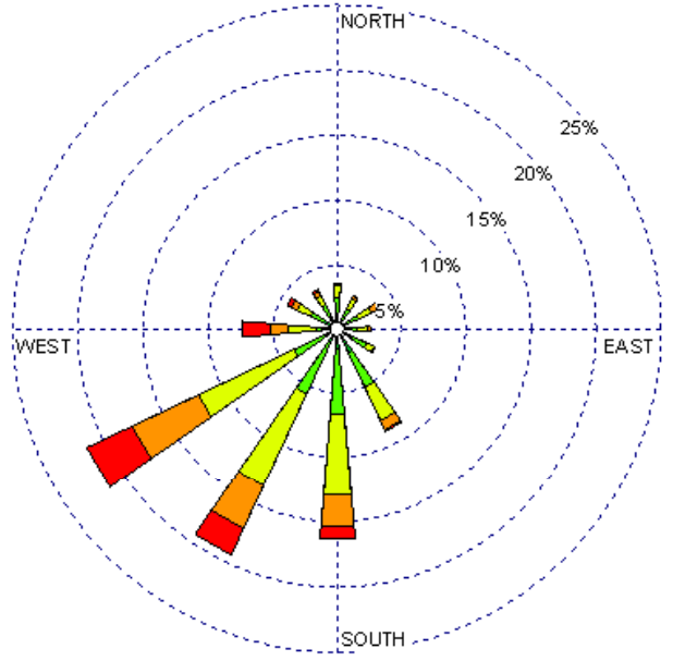
Las Vegas (23054) 1985-2005 May - 19-23z Average Speed - 13.43 kt
