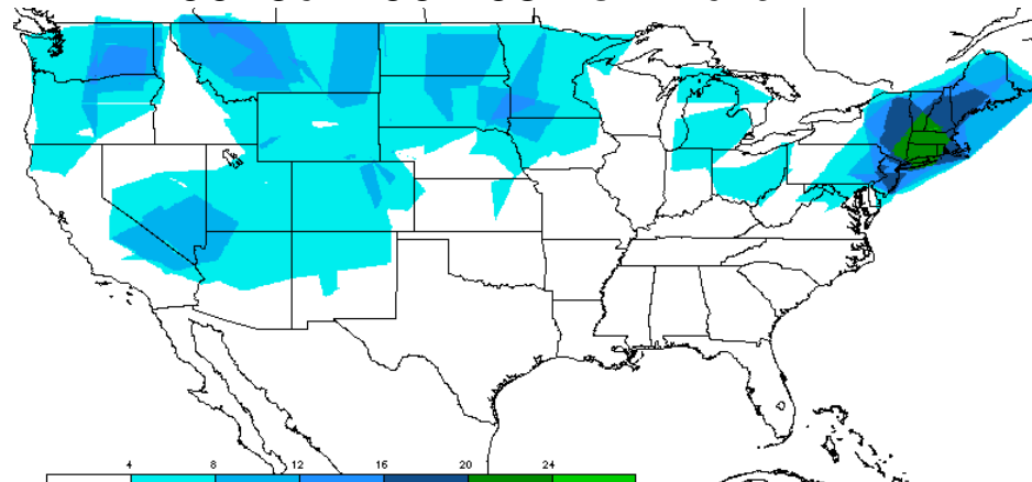
00ZJul 2001-03 IFR
