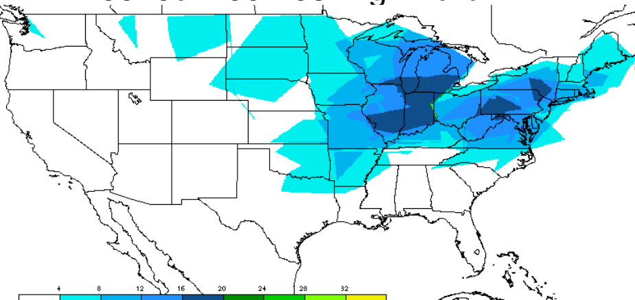
00ZJul 2001-03 Icing
